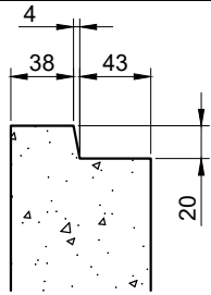
TOP REBATE
