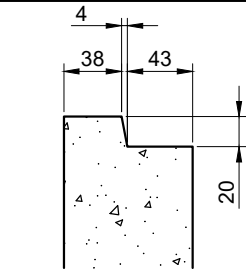
TOP REBATE
